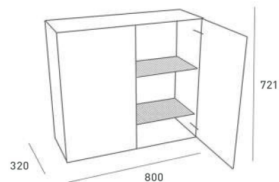
Шкаф навесной с сушкой
