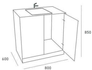
Стол с мойкой
